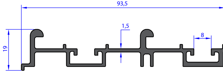
AU 71190 WEIGHT 0.873 Kg/m
