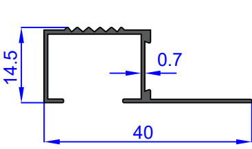
AU 72336 WEIGHT 0.158 Kg/m
