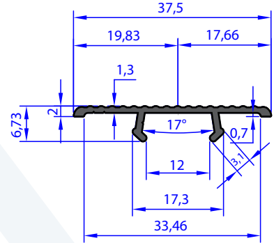
A.3210 WEIGHT 0.159 Kg/m
