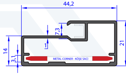
AU 71887 WEIGHT 0.437 Kg/m
