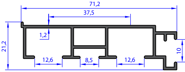
AU 72309 WEIGHT 0.591 Kg/m
