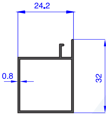
AU 71066 WEIGHT 0.249 Kg/m
