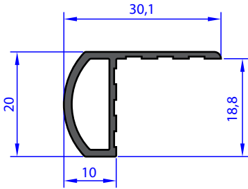
A.3123 WEIGHT 0.238 Kg/m
