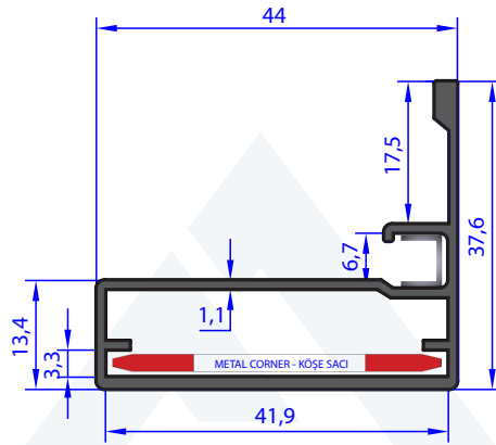
A.3096 WEIGHT 0.517 Kg/m
