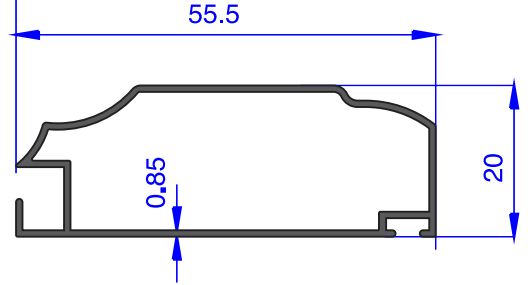
AU 71065 WEIGHT 0.353 Kg/m
