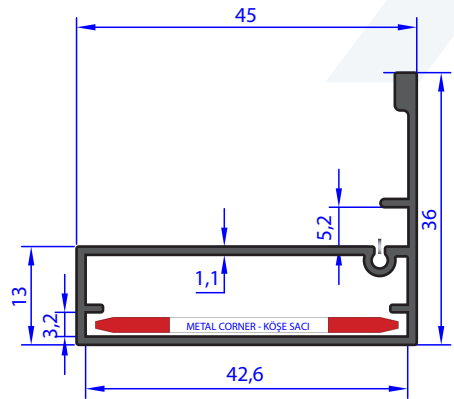
AU 72202 WEIGHT 0.469 Kg/m
