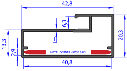
AU 71104 WEIGHT 0.385 Kg/m
