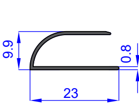
AU 72284 WEIGHT 0.104 Kg/m
