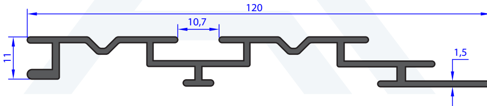
AU 71838 WEIGHT 0.889 Kg/m
