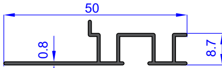
AU 72336 WEIGHT 0.158 Kg/m
