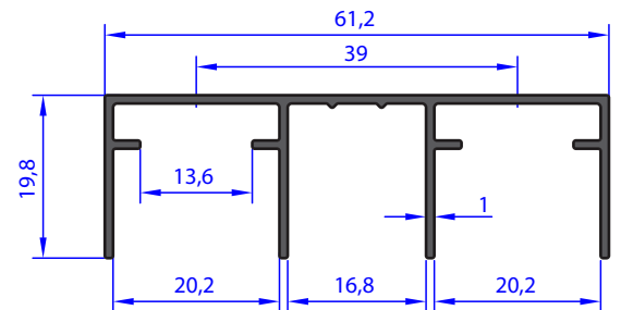
AB 96795 WEIGHT 0.407 Kg/m
