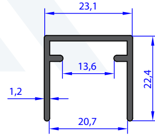
A.3035 WEIGHT 0.231 Kg/m
