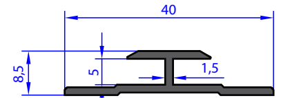
AB 92829 WEIGHT 0.243 Kg/m
