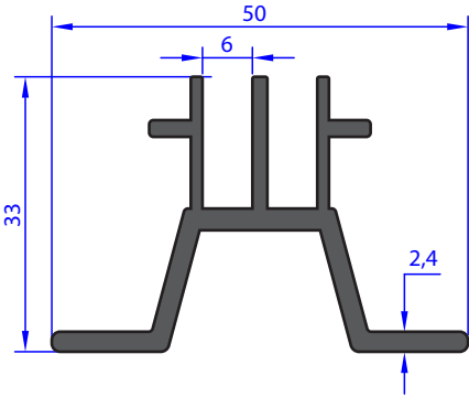
AU 71005 WEIGHT 0.729 Kg/m
