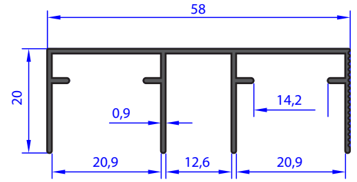
AU 72639 WEIGHT 0.356 Kg/m
