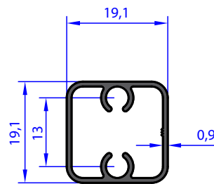
AB 97771 WEIGHT 0.224 Kg/m
