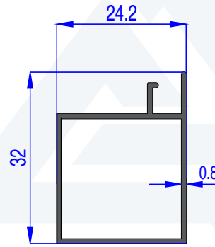
AU 71863 WEIGHT 0.249 Kg/m
