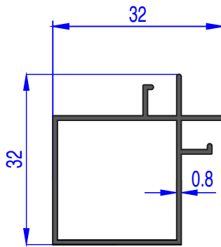
AU 71864 WEIGHT 0.282 Kg/m
