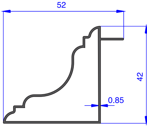
AU 71064 WEIGHT 0.368 Kg/m
