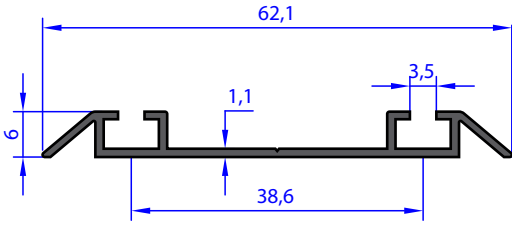
AB 95208 WEIGHT 0.269 Kg/m
