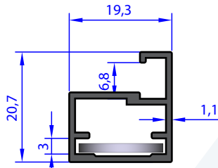
AU 72307 WEIGHT 0.253 Kg/m
