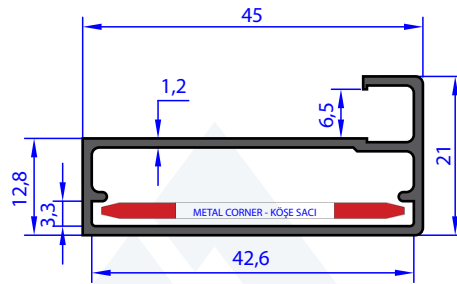
AB 96778 WEIGHT 0.426 Kg/m
