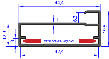
AU 72746 WEIGHT 0.372 Kg/m
