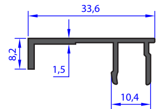
AU 71801 WEIGHT 0.223 Kg/m
