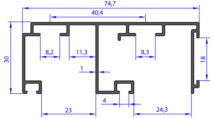
AU 71983 WEIGHT 0.659 Kg/m
