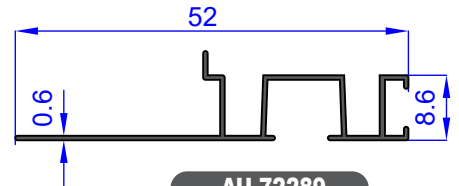
AU 72289 WEIGHT 0.160 Kg/m
