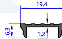
AB 92837 WEIGHT 0.106 Kg/m
