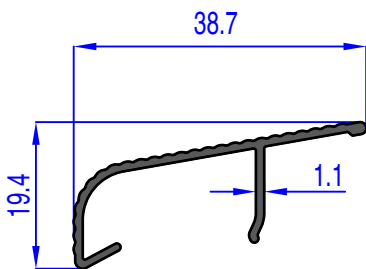
AU 71828 WEIGHT 0.201 Kg/m
