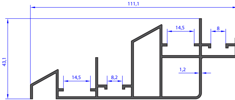
AU 71273 WEIGHT 1.128 Kg/m
