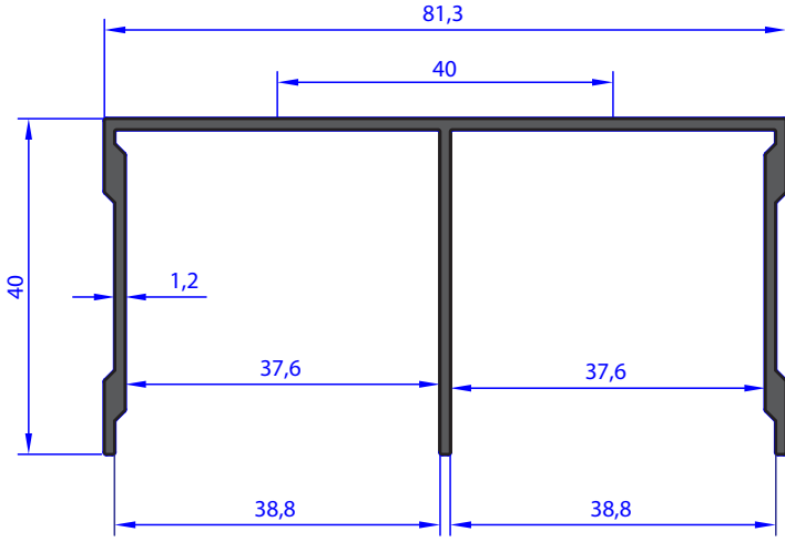
AU 73162 WEIGHT 0.738 Kg/m
