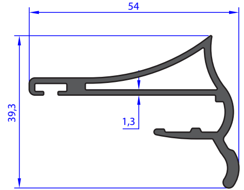
AU 72737 WEIGHT 0.689 Kg/m
