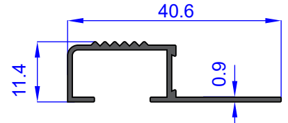
AU 72024 WEIGHT 0.181 Kg/m
