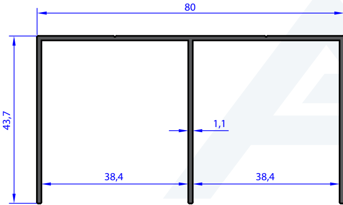
AU 73092 WEIGHT 0.621 Kg/m
