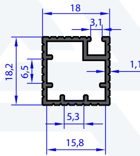
AU 73025 WEIGHT 0.234 Kg/m
