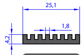
AB 95016 WEIGHT 0.223 Kg/m
