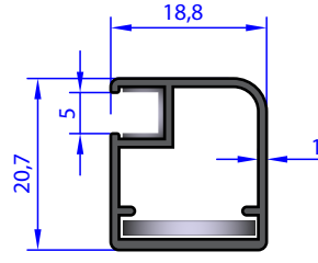
AU 71105 WEIGHT 0.244 Kg/m
