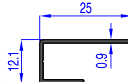
AU 72793 WEIGHT 0.116 Kg/m
