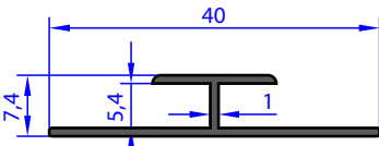
AB 92703 WEIGHT 0.162 Kg/m
