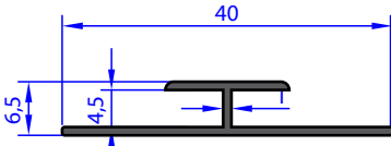
AB 92764 WEIGHT 0.160 Kg/m
