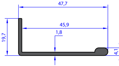
AU 72840 WEIGHT 0.356 Kg/m
