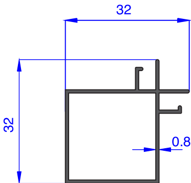
AU 71068 WEIGHT 0.282 Kg/m
