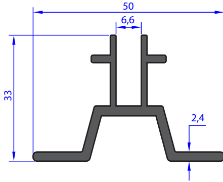
AU 71003 WEIGHT 0.655 Kg/m
