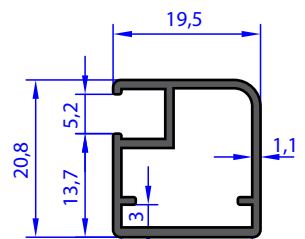
AU 71037 WEIGHT 0.269 Kg/m
