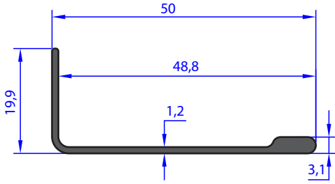
AU 72869 WEIGHT 0.261 Kg/m
