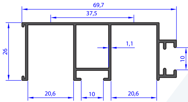
AU 72344 WEIGHT 0.613 Kg/m
