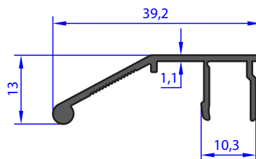
AU 72308 WEIGHT 0.225 Kg/m
