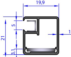
AU 71888 WEIGHT 0.261 Kg/m
