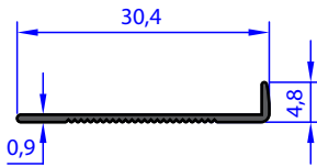
AU 72969 WEIGHT 0.079 Kg/m
