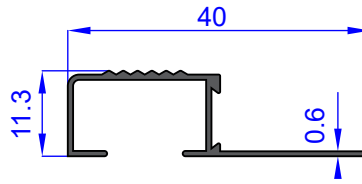
AU 72285 WEIGHT 0.143 Kg/m
