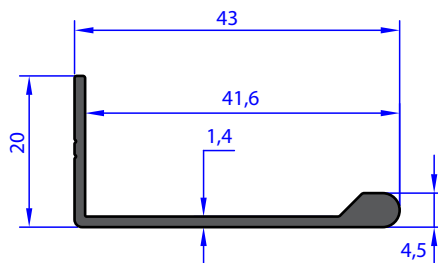
AU 72900 WEIGHT 0.288 Kg/m
