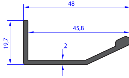
AU 72832 WEIGHT 0.404 Kg/m
