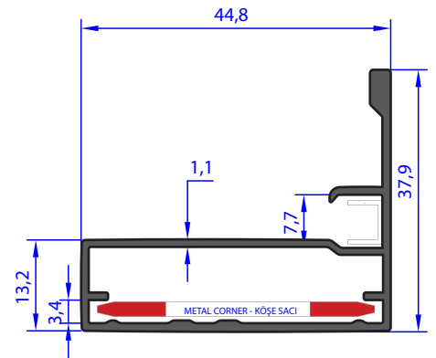
AU 71821 WEIGHT 0.499 Kg/m
