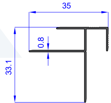
AU 72290 WEIGHT 0.190 Kg/m
