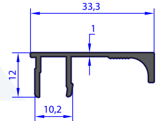
AB 92622 WEIGHT 0.224 Kg/m
