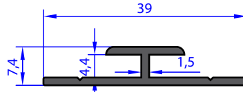
AB 95316 WEIGHT 0.235 Kg/m
