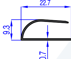
AU 72735 WEIGHT 0.093 Kg/m
