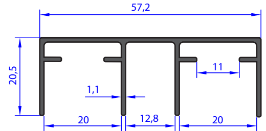
AU 71868 WEIGHT 0.814 Kg/m
