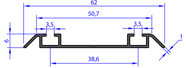
AU 72966 WEIGHT 0.255 Kg/m
