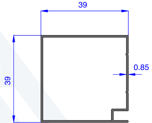
AU 71067 WEIGHT 0.367 Kg/m
