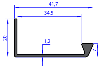
AU 73073 WEIGHT 0.261 Kg/m
