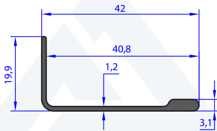
AU 72687 WEIGHT 0.234 Kg/m
