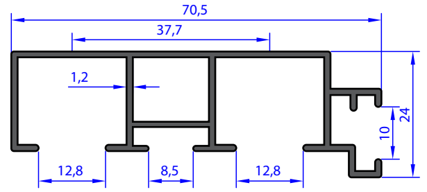
AU 72426 WEIGHT 0.624 Kg/m
