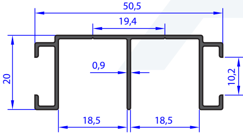
AU 72001 WEIGHT 0.320 Kg/m
