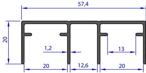
AU 71060 WEIGHT 0.467 Kg/m
