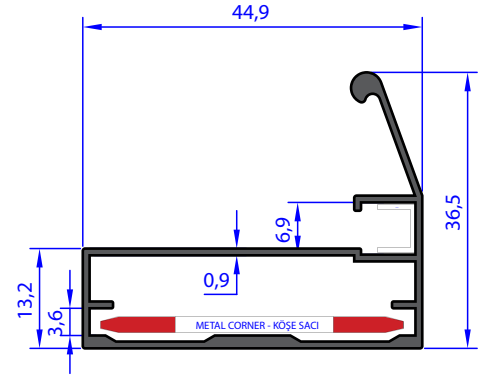
AU 72681 WEIGHT 0.437 Kg/m
