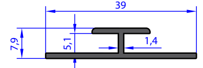
AB 95143 WEIGHT 0.223 Kg/m
