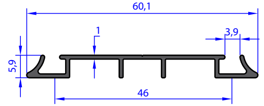
AB 92232 WEIGHT 0.268 Kg/m
