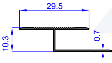
AU 72287 WEIGHT 0.120 Kg/m
