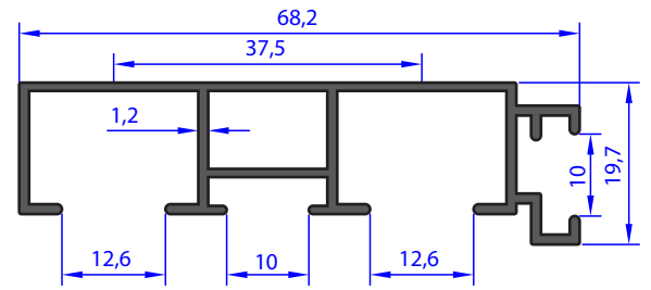
AU 72345 WEIGHT 0.551 Kg/m
