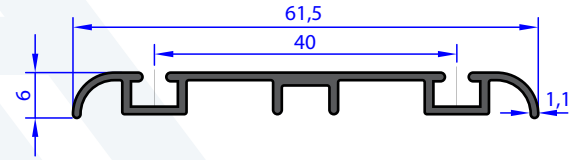
AU 71281 WEIGHT 0.297 Kg/m
