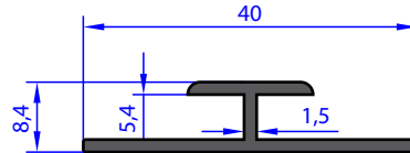
AB 92549 WEIGHT 0.251 Kg/m
