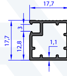
AB 96487 WEIGHT 0.222 Kg/m
