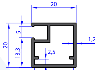
AU 71105 WEIGHT 0.244 Kg/m
