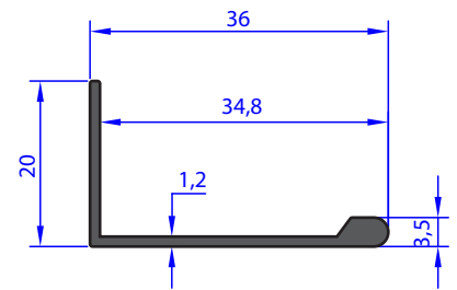
AU 72814 WEIGHT 0.209 Kg/m
