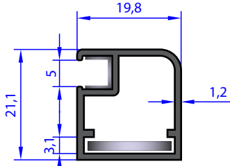
AU 72199 WEIGHT 0.288 Kg/m
