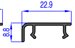
AU 71829 WEIGHT 0.129 Kg/m
