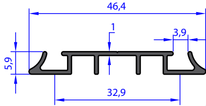
AB 92231 WEIGHT 0.223 Kg/m
