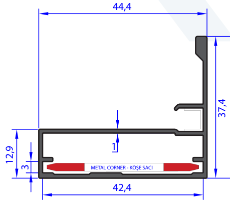
AU 72745 WEIGHT 0.450 Kg/m
