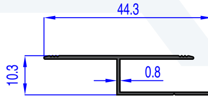
AU 72735 WEIGHT 0.093 Kg/m
