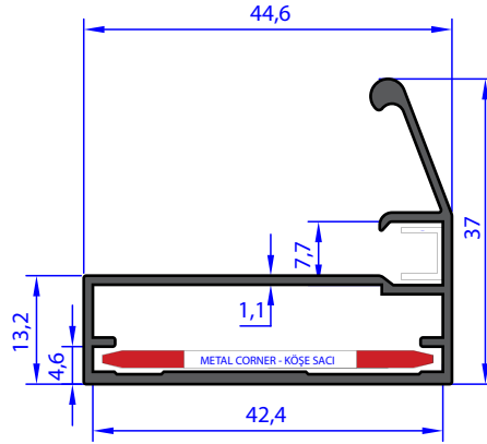
AU 72585 WEIGHT 0.499 Kg/m
