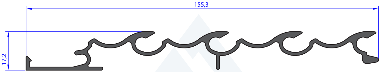
AU 72589 WEIGHT 1.1161 Kg/m
