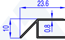
AU 72568 WEIGHT 0.112 Kg/m
