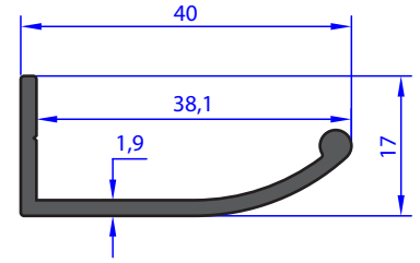
AU 72859 WEIGHT 0.309 Kg/m
