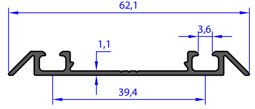
AB 97185 WEIGHT 0.287 Kg/m
