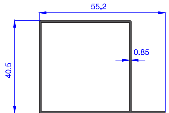
AU 71069 WEIGHT 0.398 Kg/m
